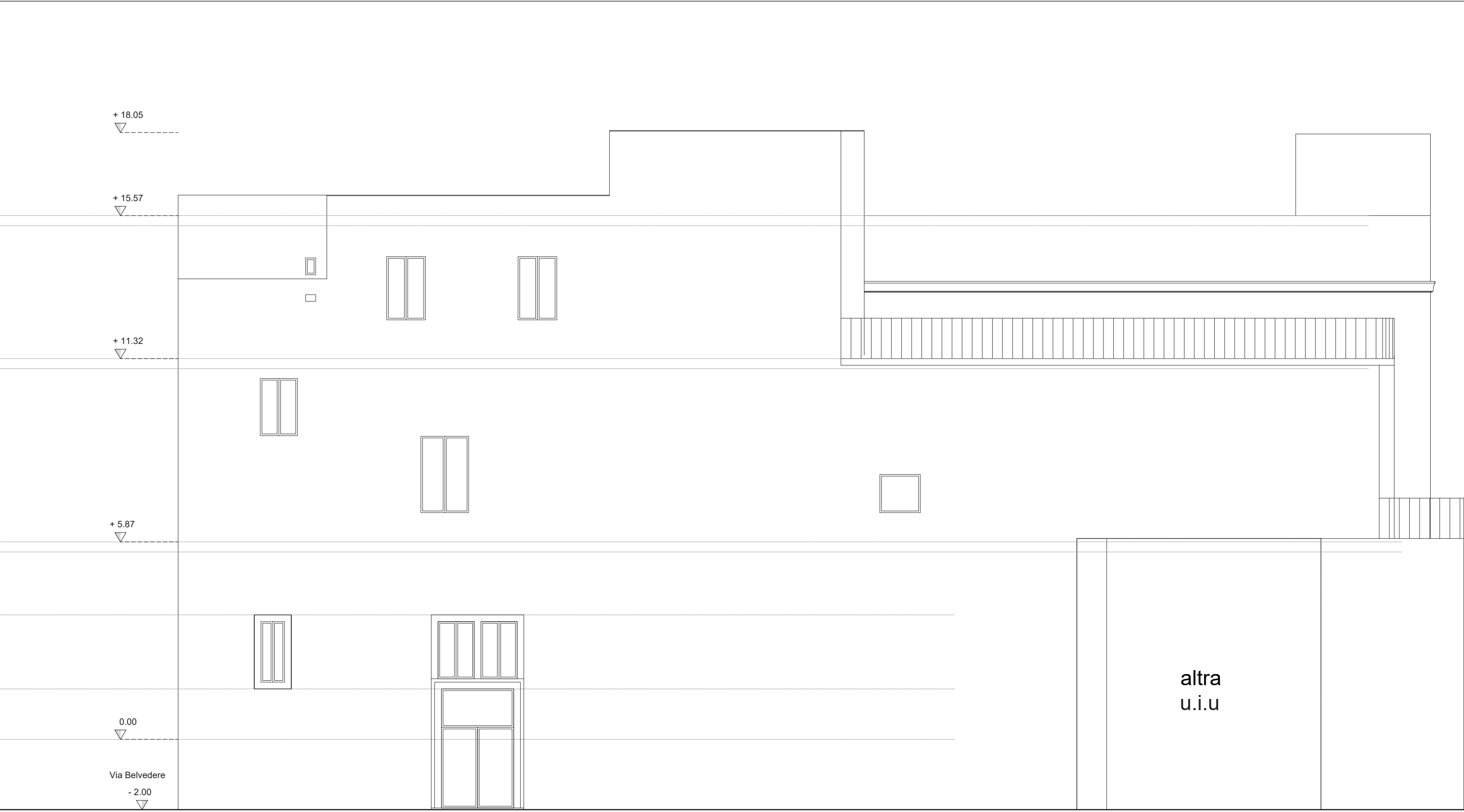
PROSPETTO VIC. BELVEDERE STATO DI FATTO - PROGETTO
