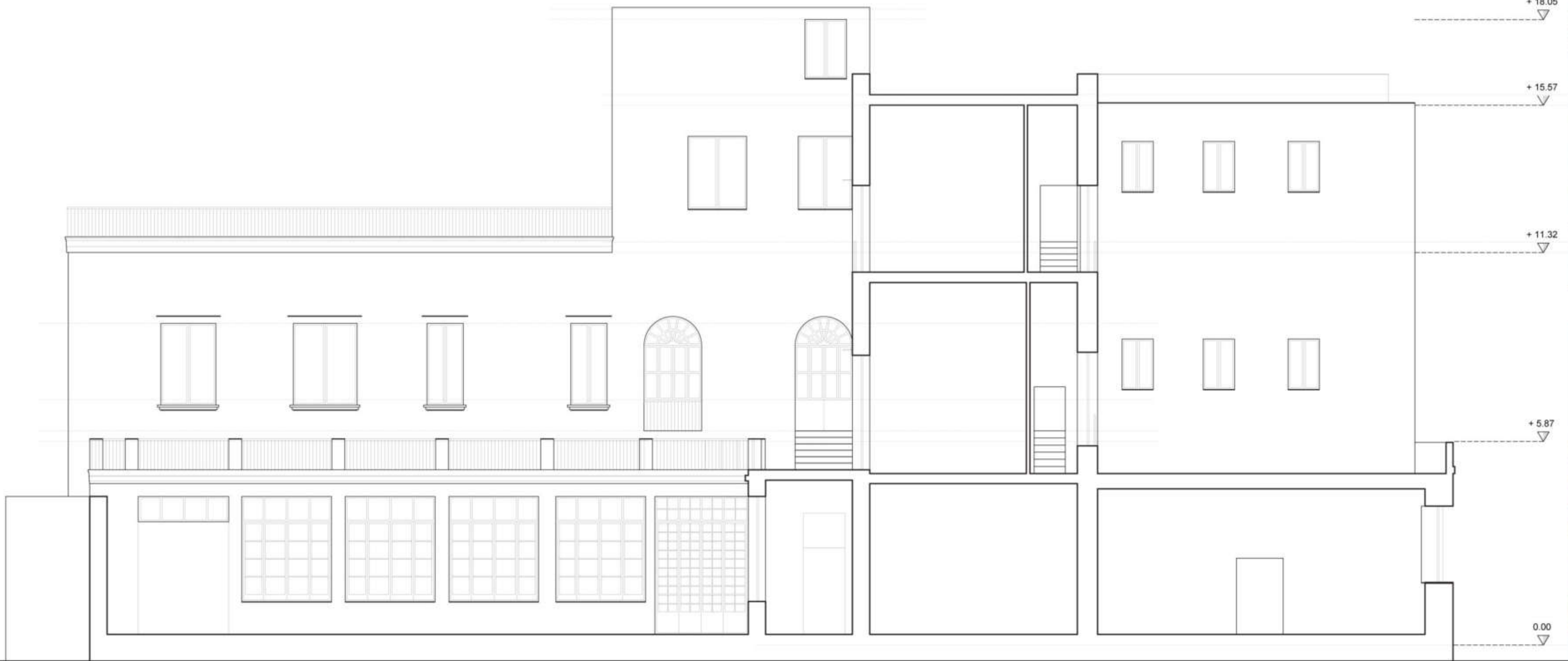
PROSPETTO-SEZ. LATO OVEST PROGETTO
