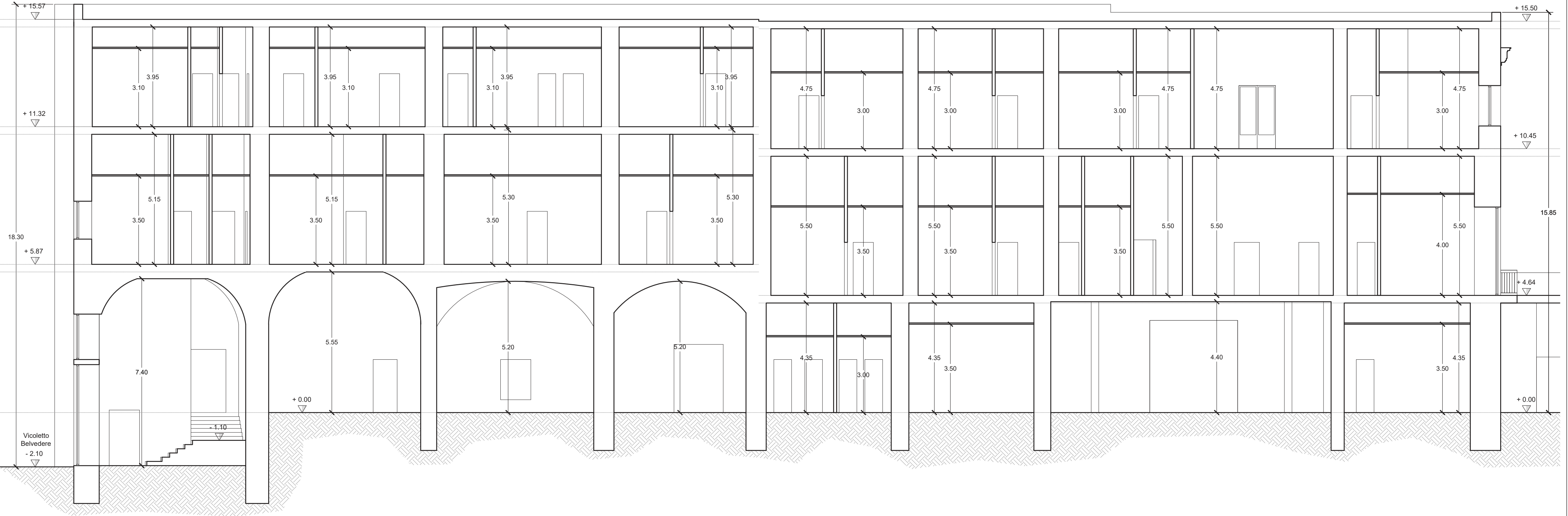
SEZIONE B - B' PROGETTO
