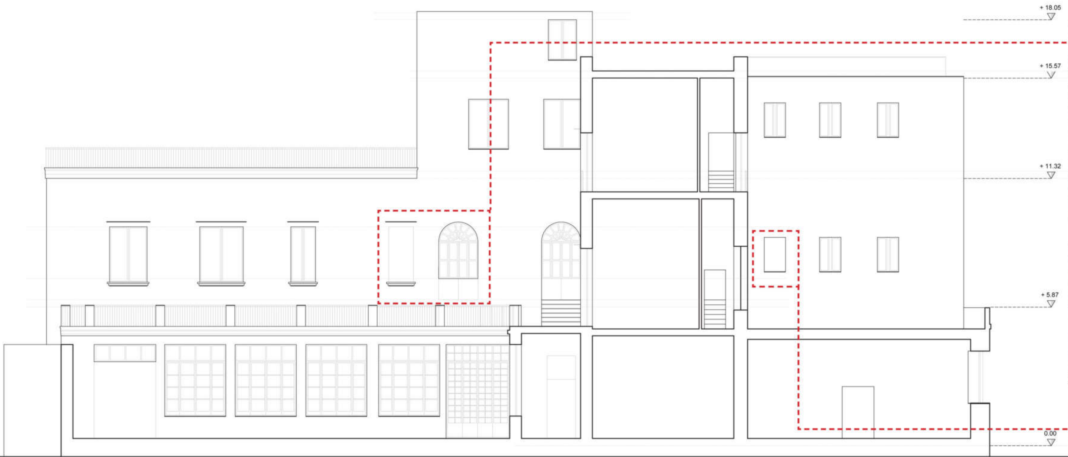
PROSPETTO-SEZ. LATO OVEST STATO DI FATTO
