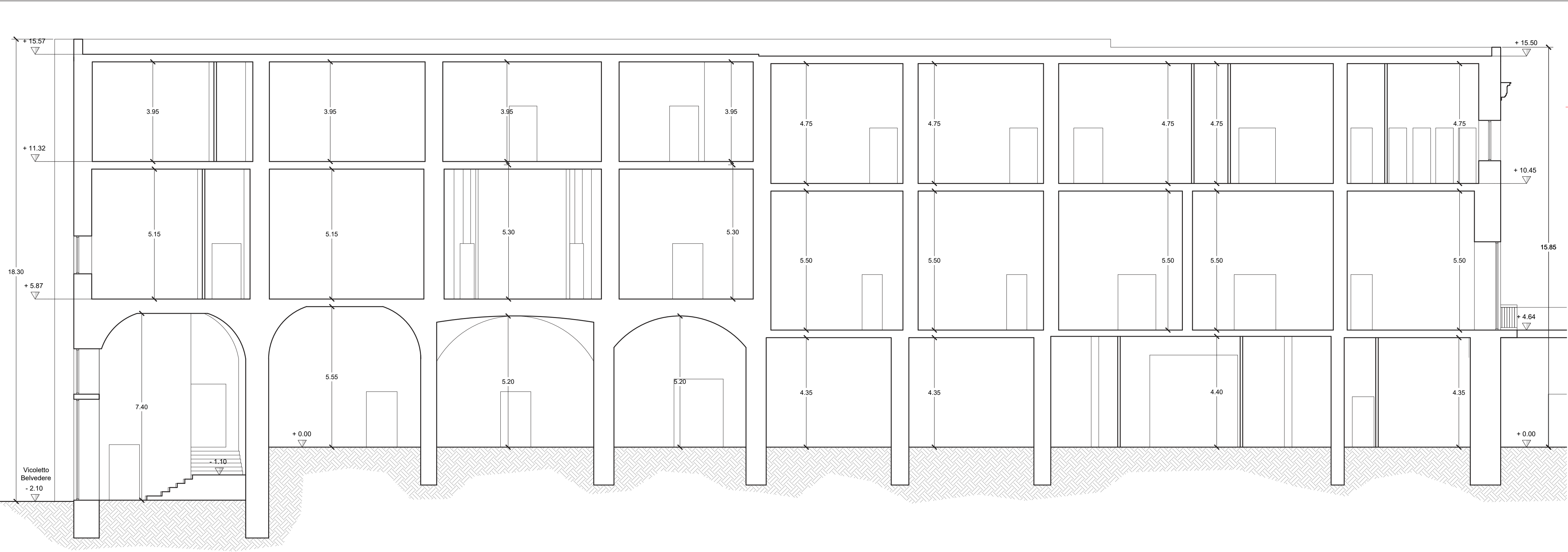
SEZIONE B - B' STATO DI FATTO
