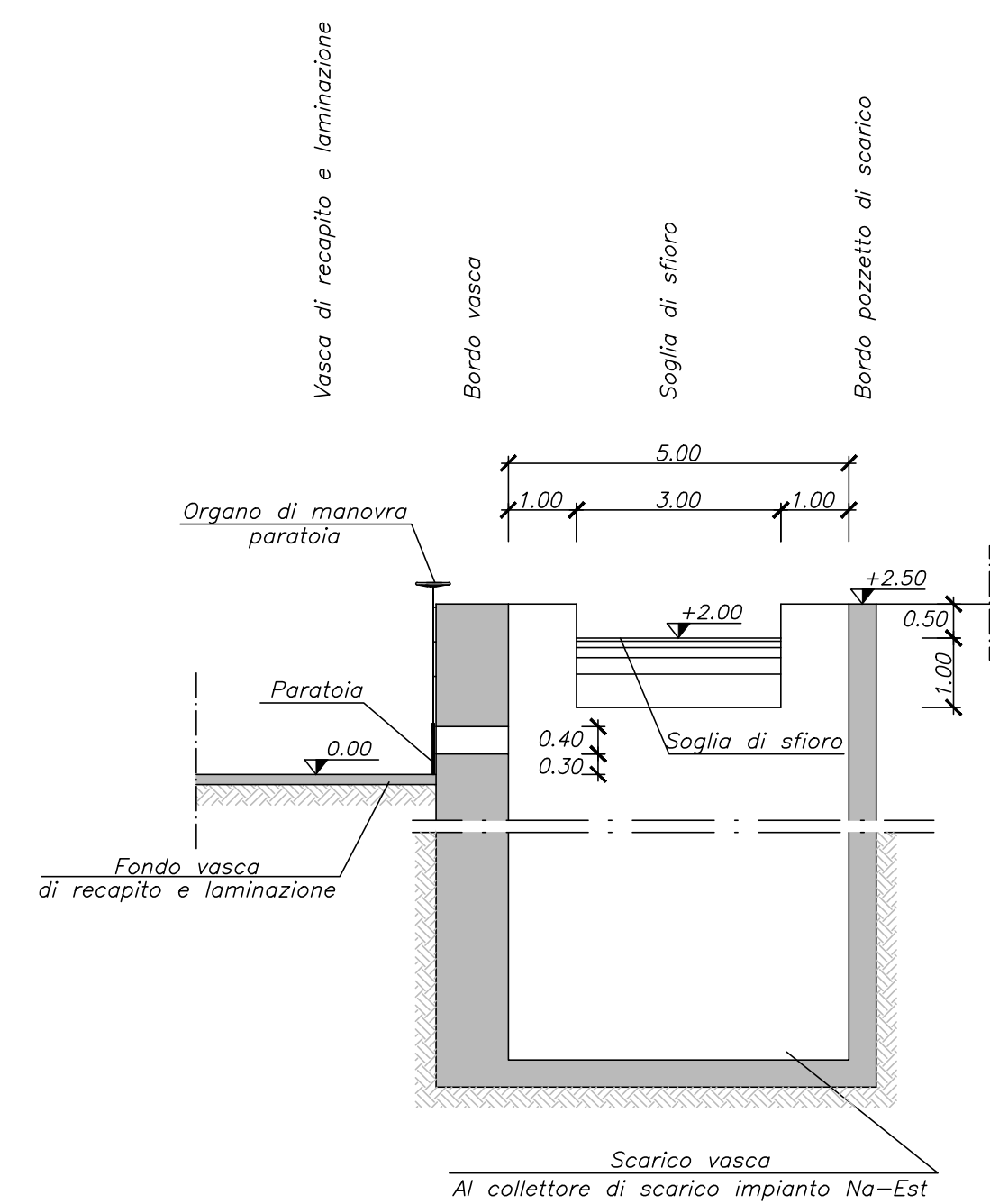
SEZIONE A-A
