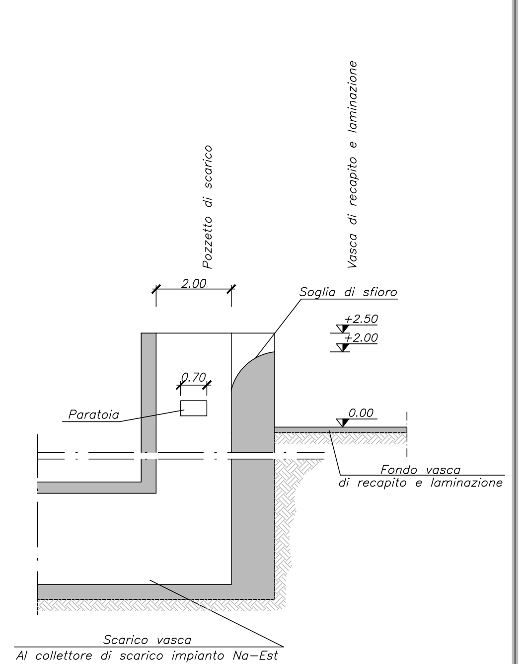
SEZIONE B-B
