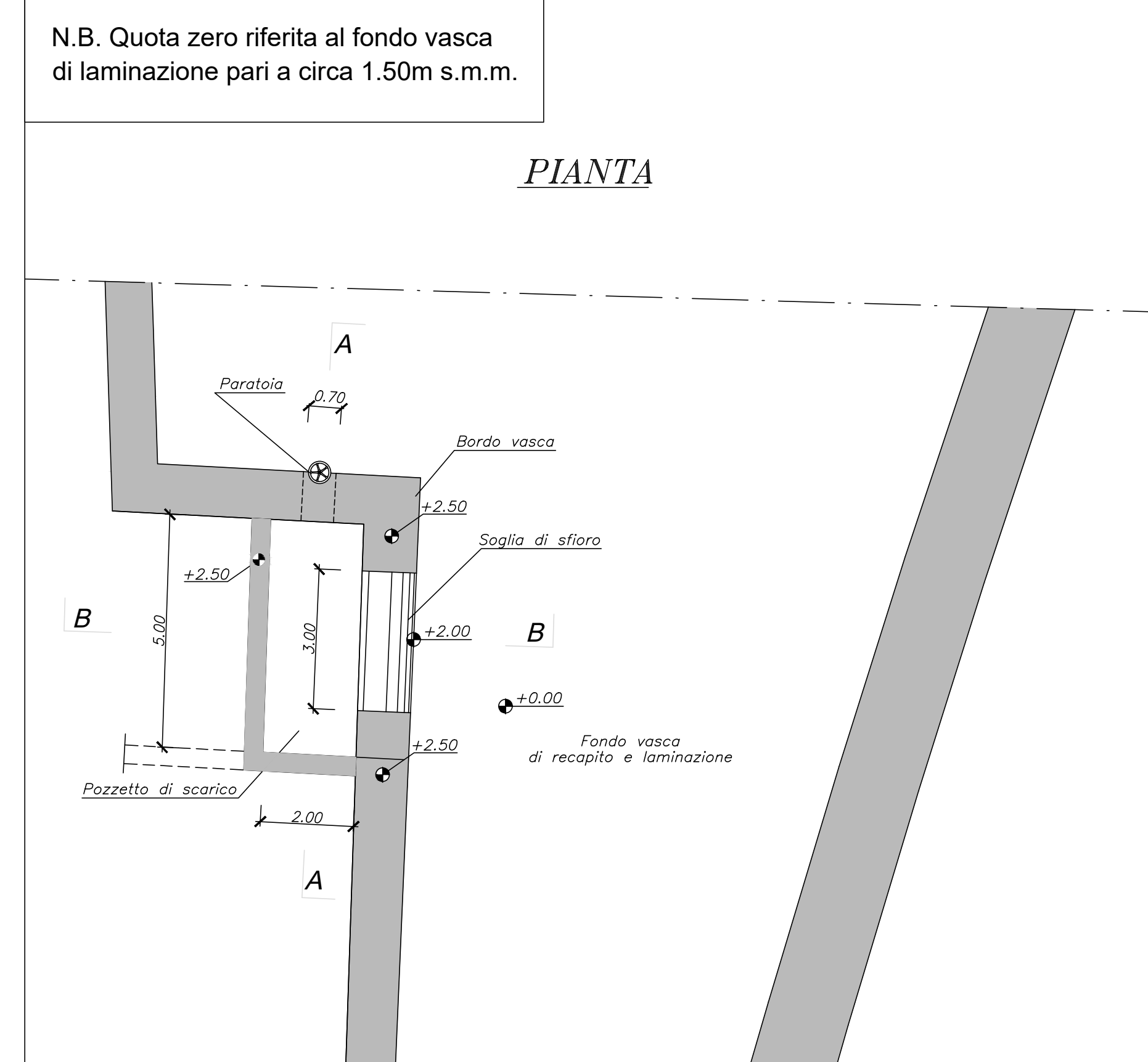
Particolare opera di scarico Scala 1:100
