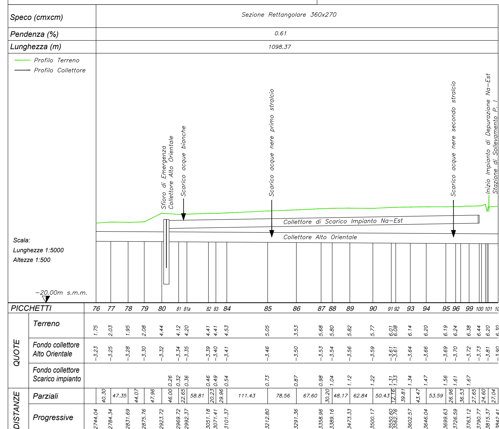
Stralcio profilo longitudinale collettori sistenti Scala 1:5000/1:500
